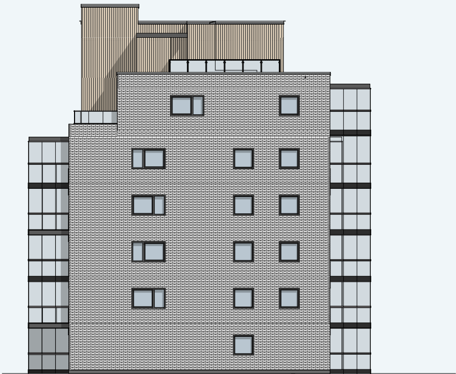
Fasade Sørvest
