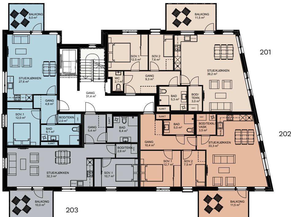
2. etasje
